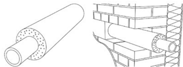
Vedení potrubí v izolaci pod omítkou
