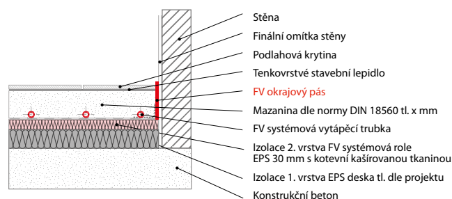
Obr. č. 10: Osazení FV okrajového pásu
