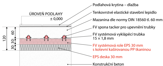
Obr. č. 17: Doporučená skladba podlahy nad rostlým terénem, místnostmi, sklepními nebo občasně vytápěnými místnostmi podle doporučení normy ČSN EN 1264 tepelný odpor izolace R = 1,25 \text{ m}^2\text{K/W}
