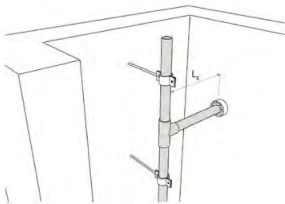
Dostatečnou vzdálenost stoupačky od prostupu stěnou
