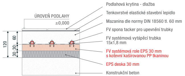
Obr. č.17: Doporučená skladba podlahy nad rostlým terémem, místnostmi, sklepními nebo občasně vytápěnými místnostmi podle doporučení normy ČSN EN 1264 tepelný odpor izolace R = 1,25 \text{ m}^2\text{K/W}
