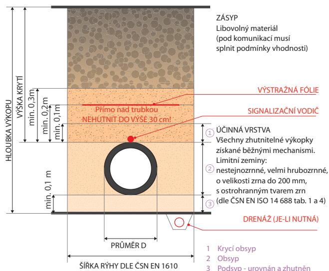
Schema uložení trubek FV HDPE 100 RC ve výkopu
