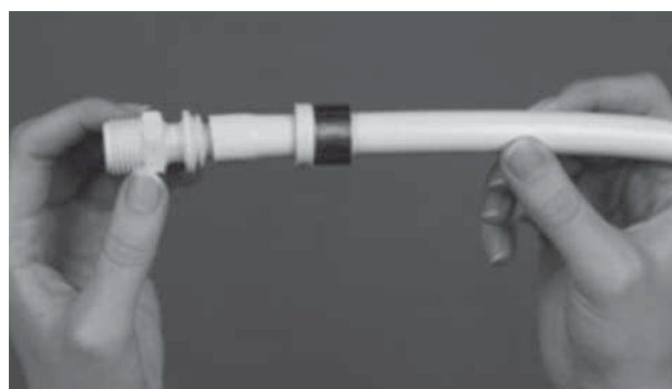
4. Vložte tvarovku do rozšířeného potrubí.
